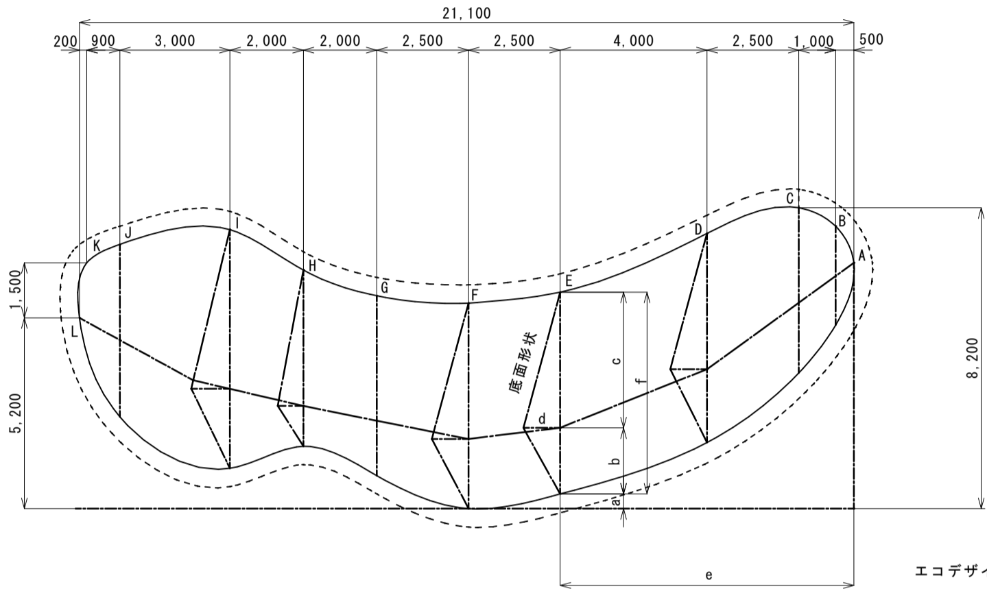
平面図
